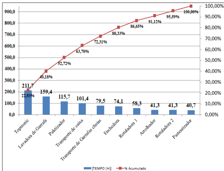
Figura 5: Gráfico com Falhas mecânicas e elétricas no ano de 2017.
