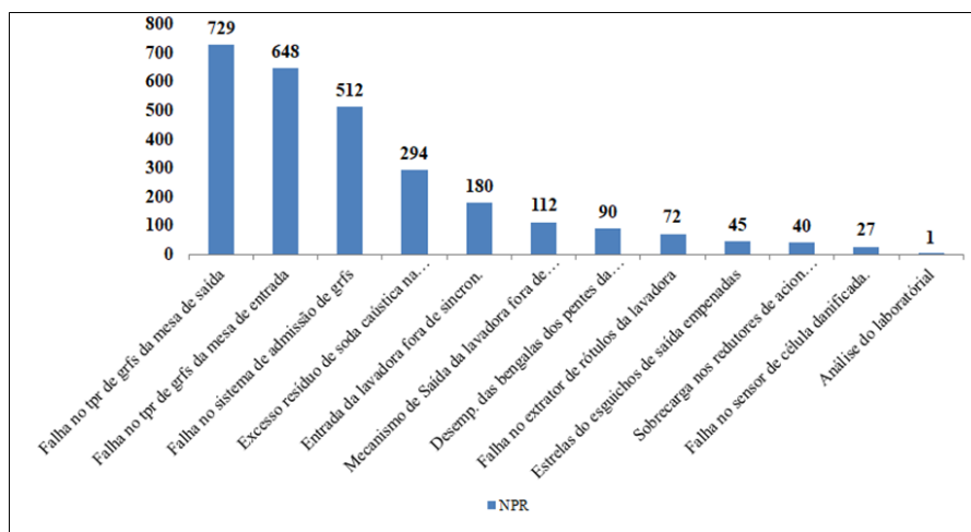
Figura 2: Gráfico com Cálculo de NPR para o grau de risco do modo de falha.
