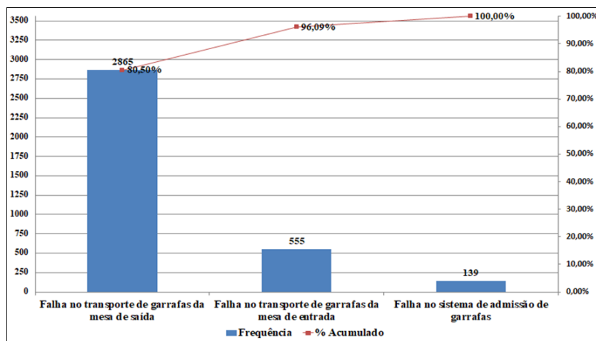
Figura 1: Diagrama de Pareto dos potenciais modos de falhas.
