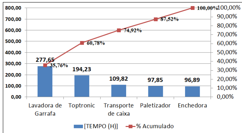
Figura 3: Gráfico das Falhas mecânicas e elétricas no ano de 2017.
